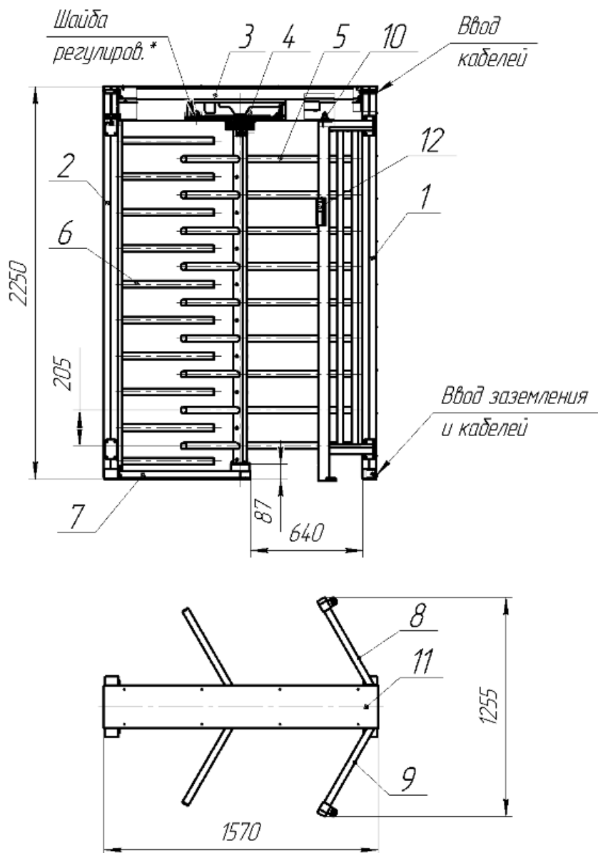
Габаритные размеры турникета «Ростов-Дон ПР1Л/ЗМ2»
